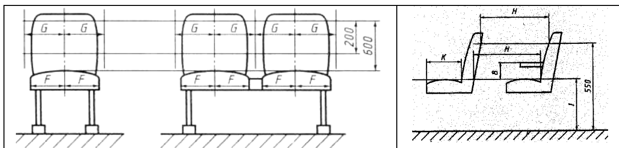
Рисунок 1.16.1. Размеры и расположение сидений
